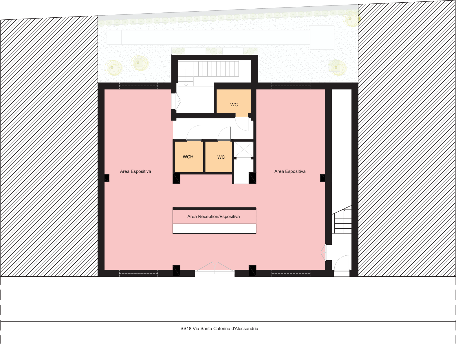
Piano terra _ Layout funzionale
