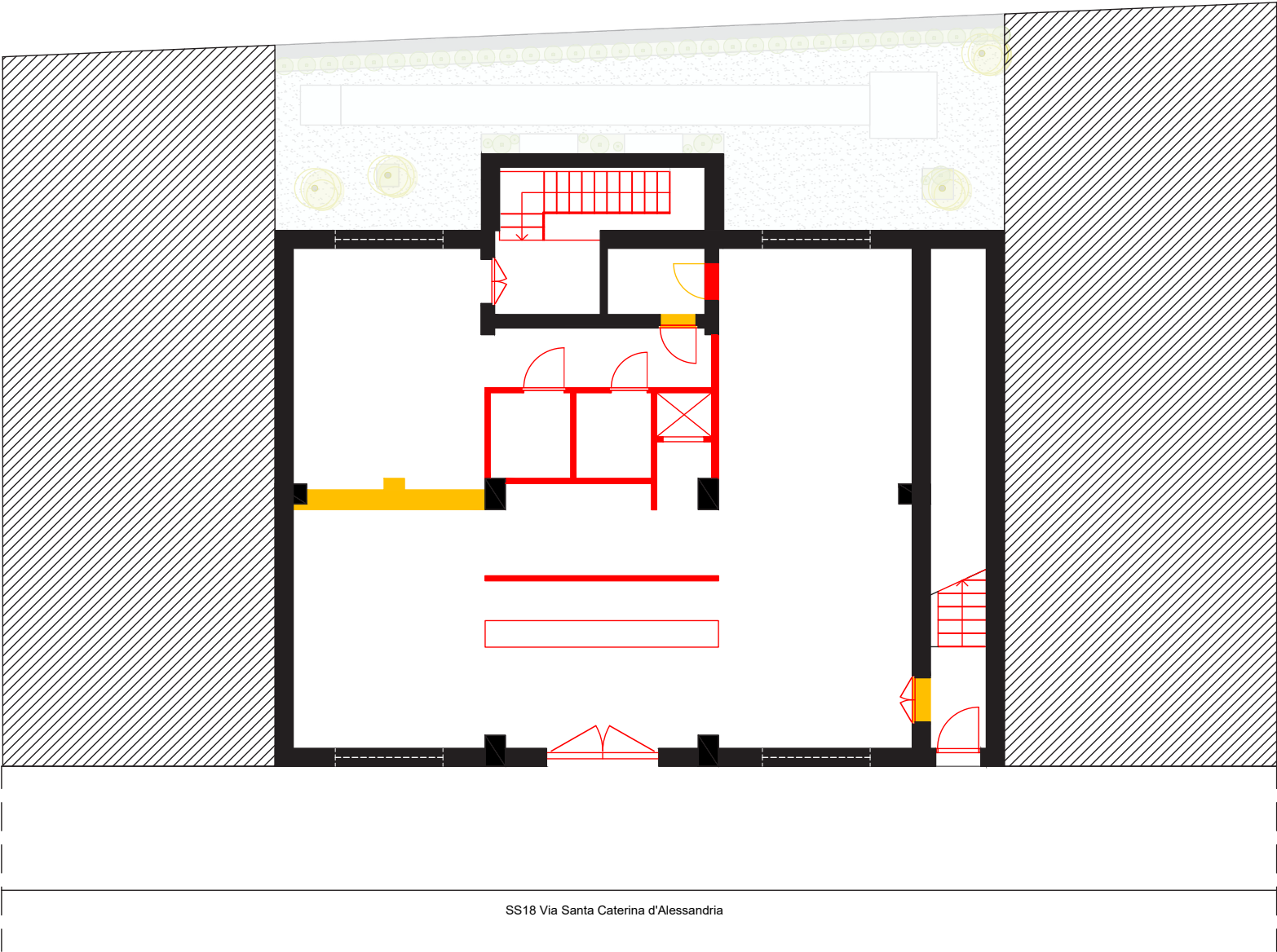
Piano terra_Raffronto Ante/Post
